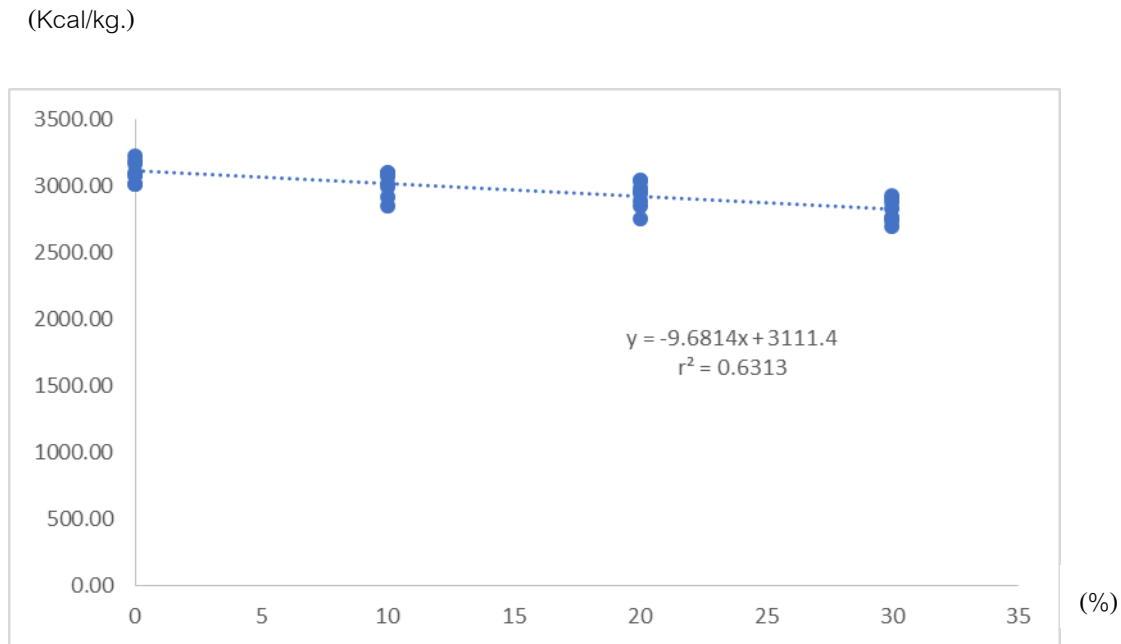
ภาพที่ 1 กราฟสมการเส้นตรงค่าพลังงาน AME ของถั่วพลอรืเกรซ
