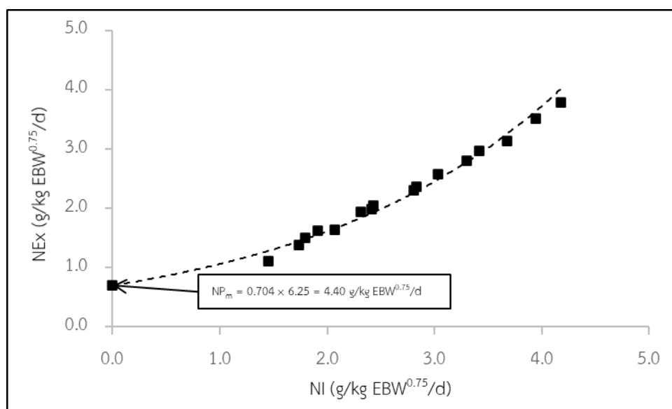
ภาพที่ 4 ความสัมพันธ์ระหว่างปริมาณการกินไนโตรเจนที่ย่อยได้ (NI) และอัตราการขับถ่ายไนโตรเจน (NEx) แสดงเป็นสมการ ดังนี้ NEx = 0.704(\pm 0.291) \times e^{(1.341(\pm 0.047) \times NI)} ( R^2=0.98 )
