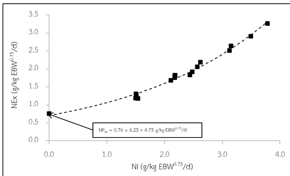
ภาพที่ 2 แสดงความสัมพันธ์ระหว่างปริมาณการกินไนโตรเจน (NI) และอัตราการขับถ่ายไนโตรเจน (NEx) โดยใช้สมการดังนี้ NEx = 0.76(\pm 0.03) \times e^{(0.39(\pm 0.01) \times NI)} ( R^2=0.99 )
